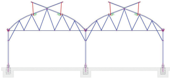
Şekil 3. Gotik Tip Makas Yapısı
